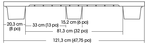
VUE DU CÔTÉ COURT
