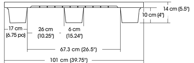
VISTA DEL LADO CORTO
