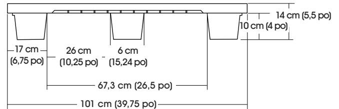
VUE DU CÔTÉ COURT
