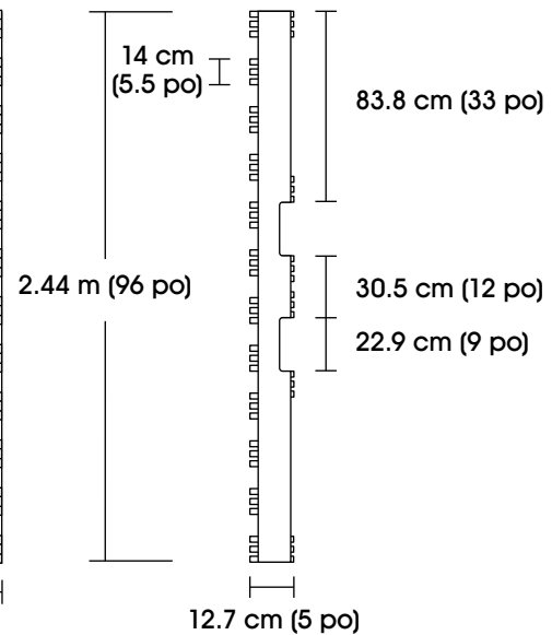
VUE LATÉRALE
