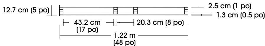
VUE D'EXTRÉMITÉ
