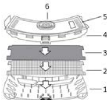
Figure 2: Como anexar o filtro/cartucho ao ventilador
