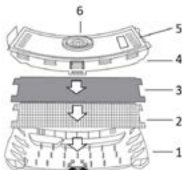
Figure 2: Fijación del filtro/cartucho al soplador
