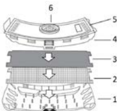
Figure 2: Fixation du filtre/cartouche au souffleur
