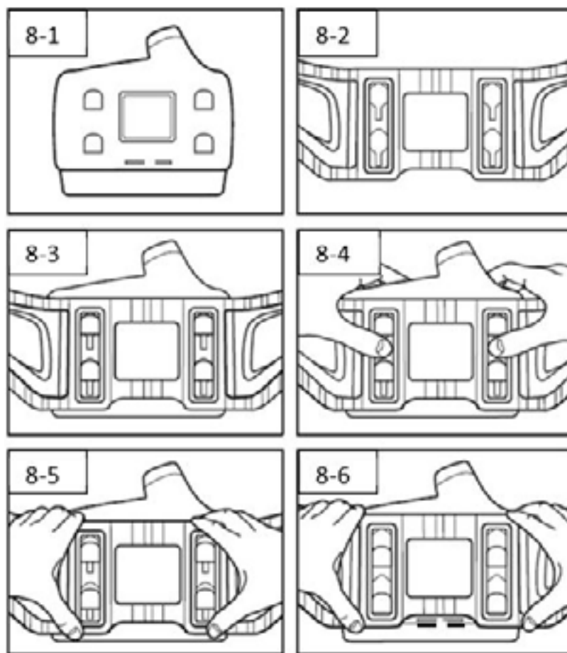
Figure 4: Instalación del cinturón
