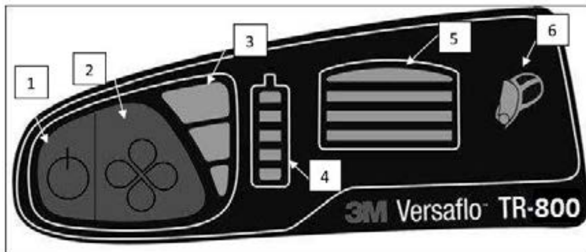
Figure 8: Interface utilisateur du souffleur à moteur : (1) Bouton marche/arrêt, (2) Bouton de régulation du débit, (3) Indicateur de réglage du débit d'air, (4) Indicateur de niveau d'état de charge de la pile/indicateur d'alarme, (5) Indicateur de charge/alarme du filtre, (6) Indicateur de mode d'ajustement serré
