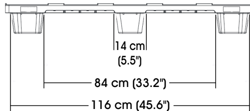
VISTA DEL LADO LARGO
