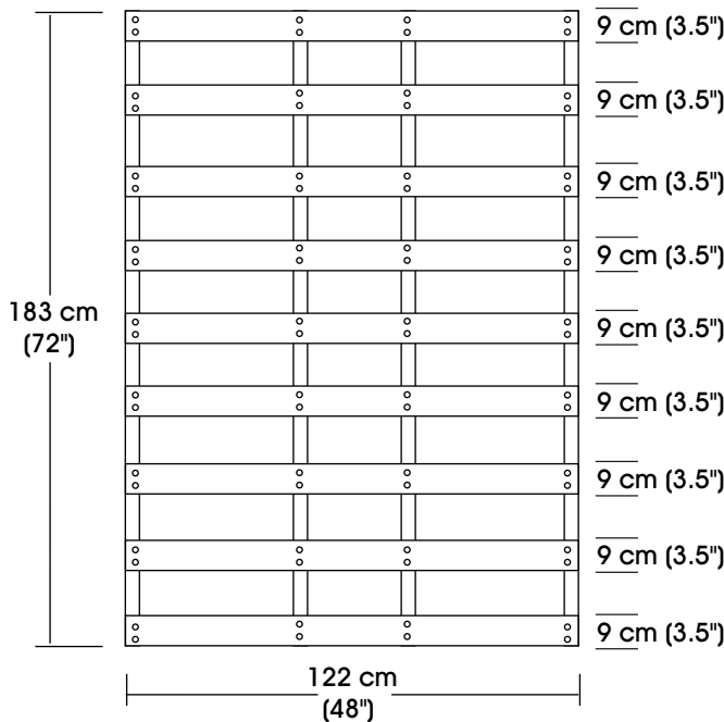
VISTA SUPERIOR
