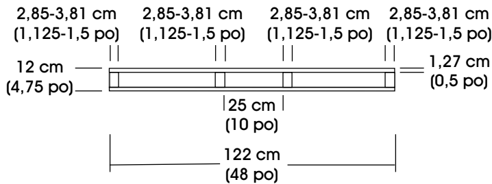
VUE LATÉRALE
