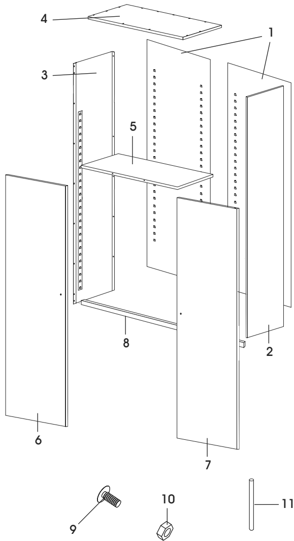
ENSAMBLE BASE
