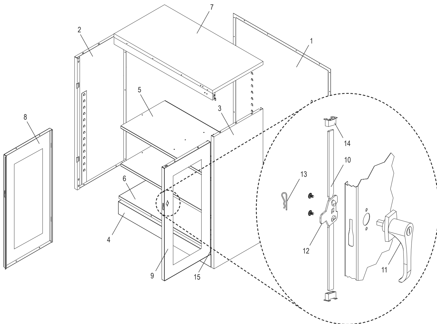
ENSAMBLE PRIMARIO
