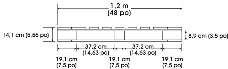
VUE LATÉRALE
