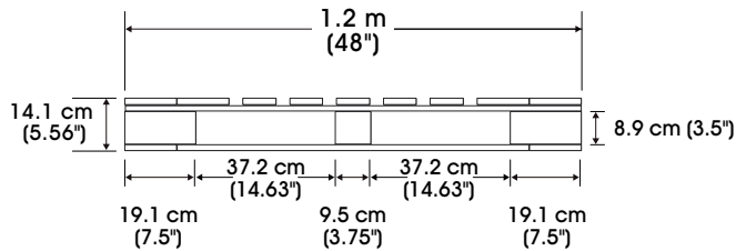
VISTA LATERAL
