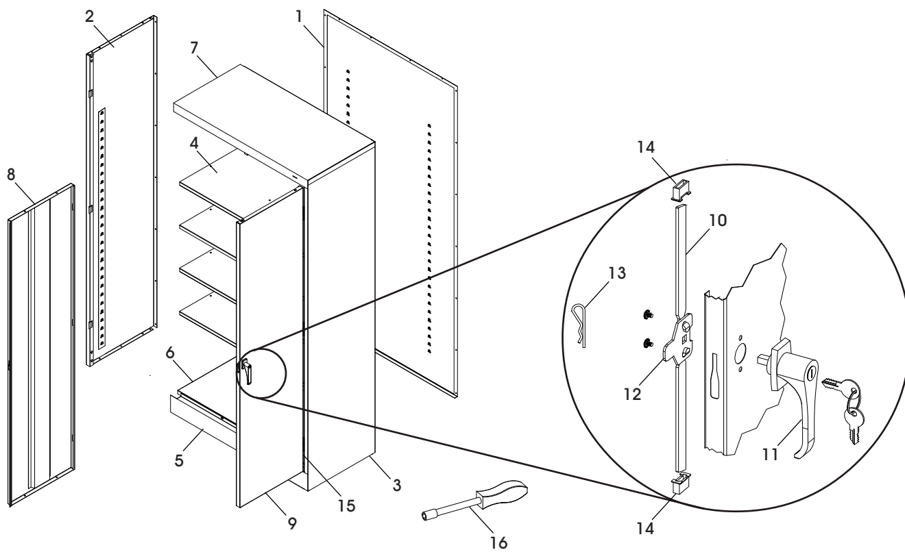
ENSEMBLE DE LA POIGNÉE
