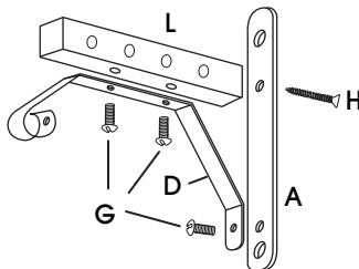
Support du milieu
