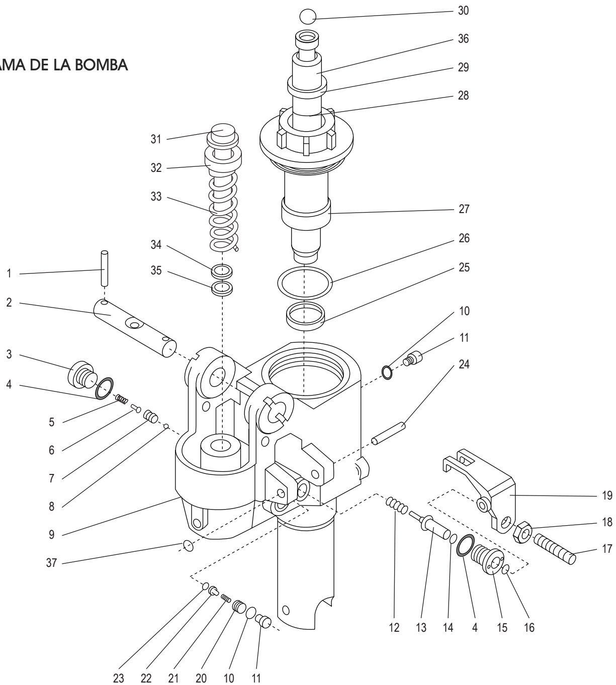
LISTA DE PARTES DEL DIAGRAMA DE LA BOMBA
