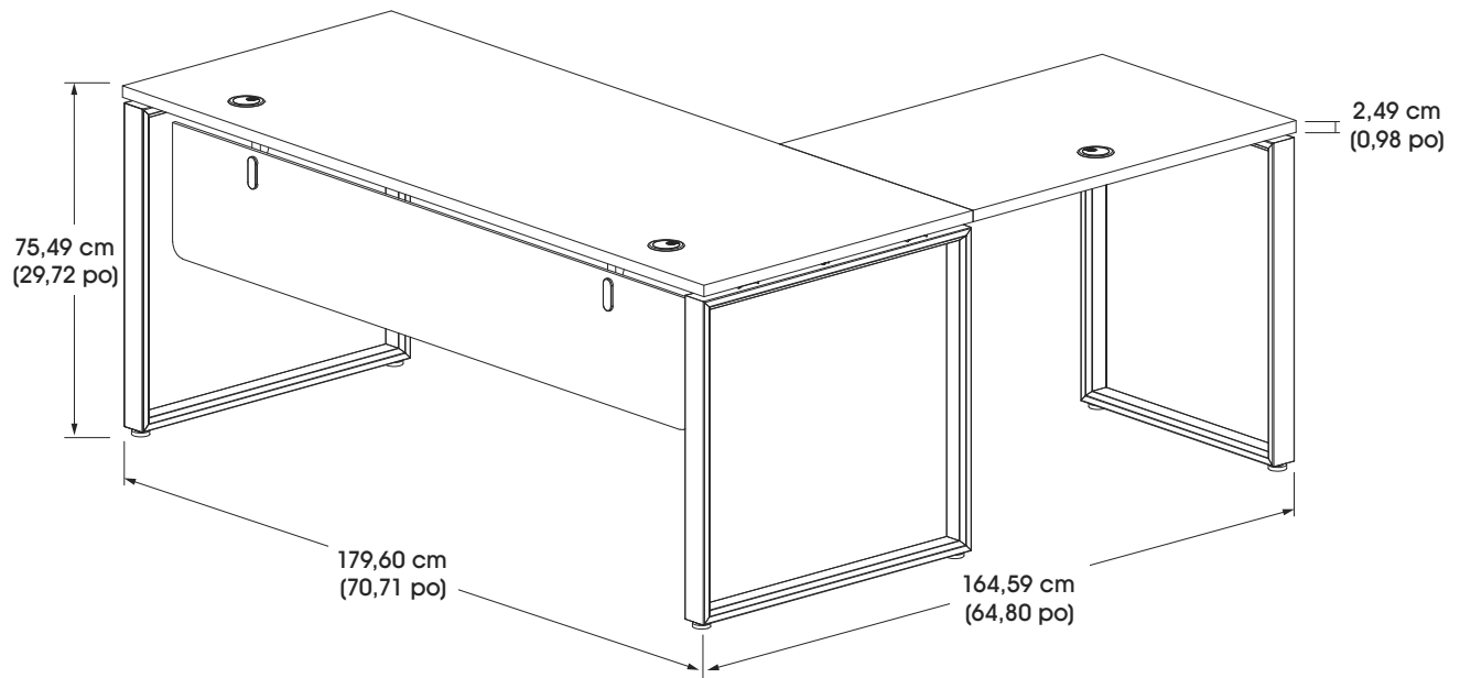
VUE INTÉRIEURE
