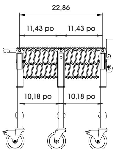
VUE LATÉRALE
