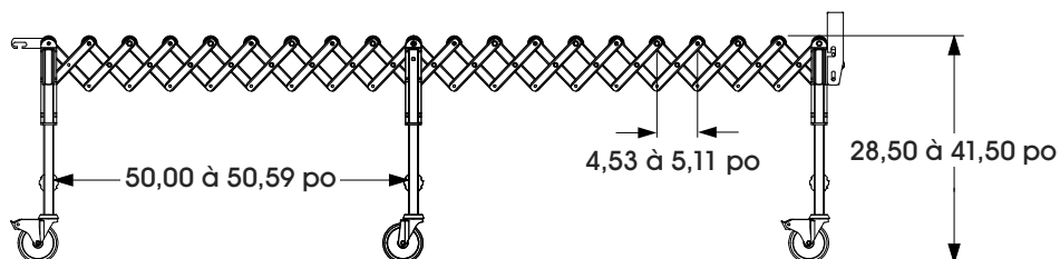
VUE LATÉRALE
