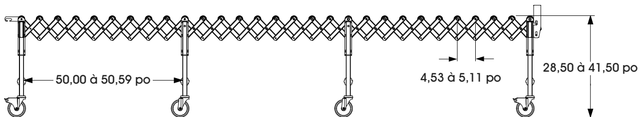
VUE LATÉRALE
