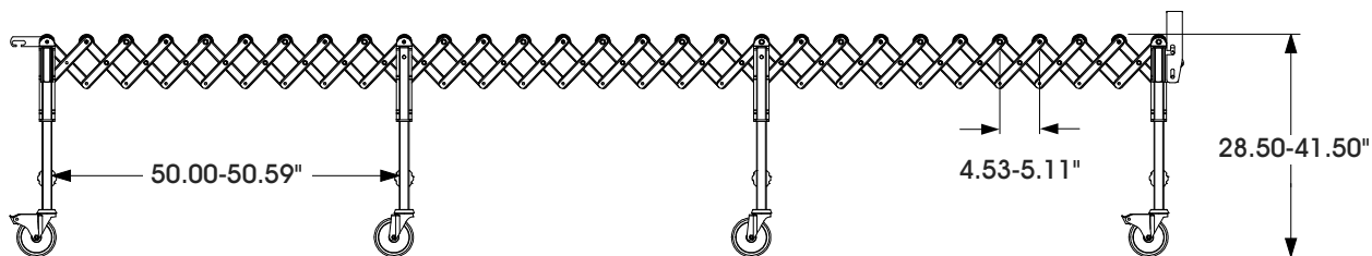
VISTA LATERAL
