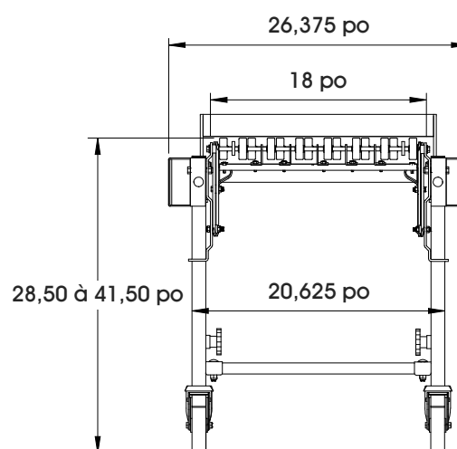
VUE D'EXTRÉMITÉ
