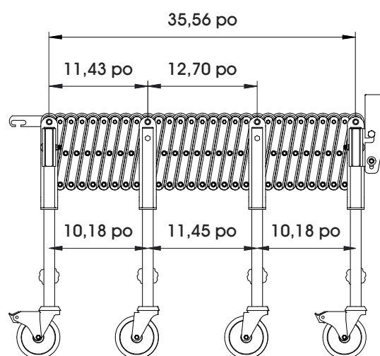
VUE LATÉRALE
