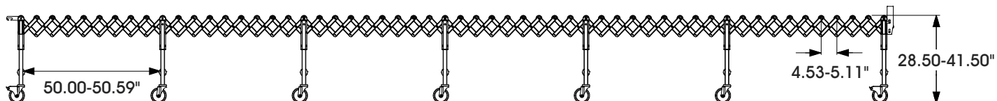
VISTA LATERAL
