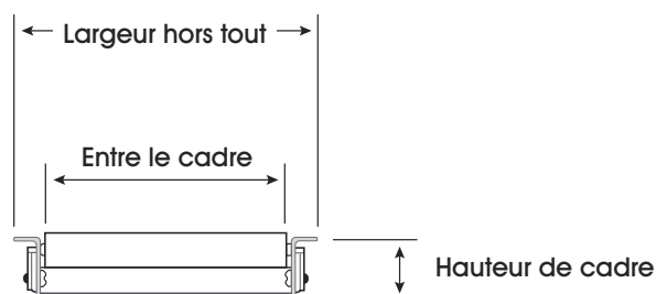
VUE LATÉRALE
