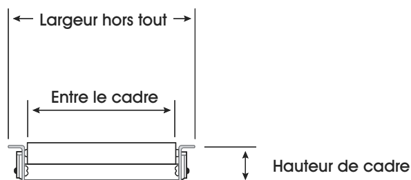
VUE LATÉRALE
