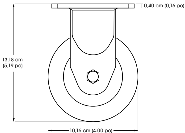
VUE LATÉRALE
