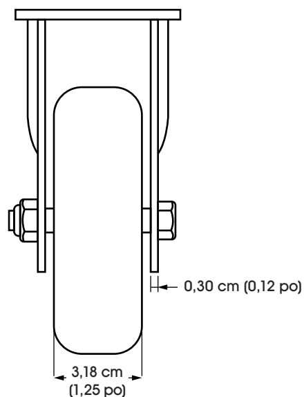
VUE AVANT
