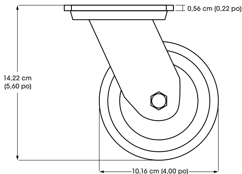
VUE LATÉRALE
