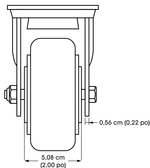
VUE AVANT
