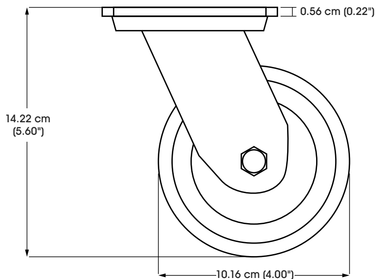
VISTA LATERAL
