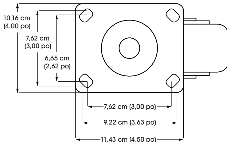
DIMENSIONS DE LA PLAQUE
