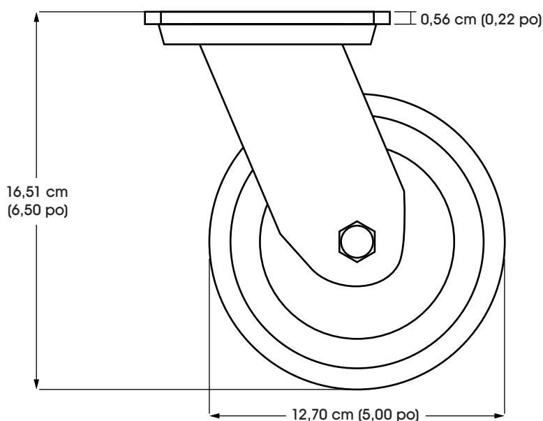
VUE LATÉRALE
