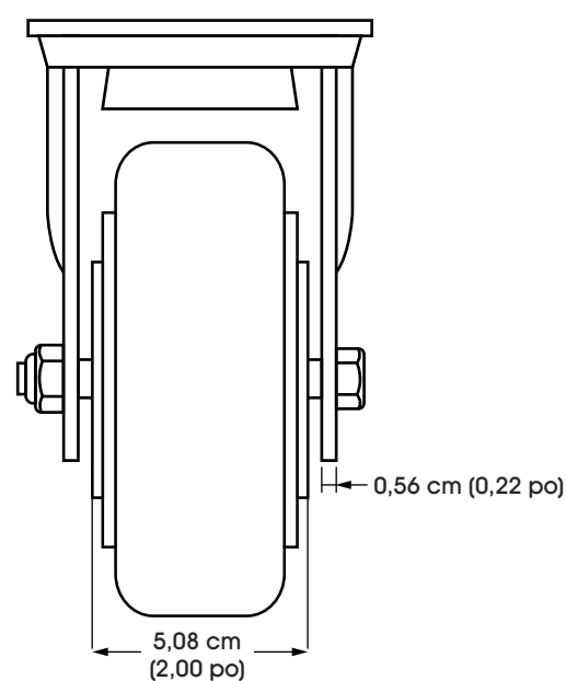
VUE AVANT
