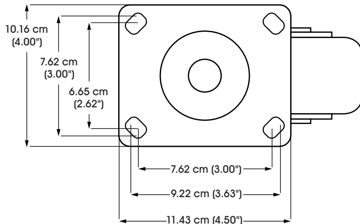
DIMENSIONES DE LA PLACA
