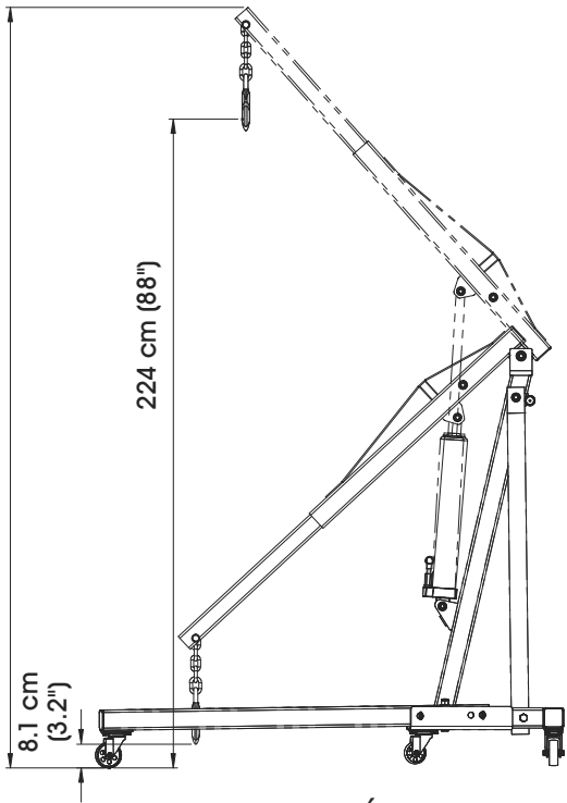
ELEVACIÓN
