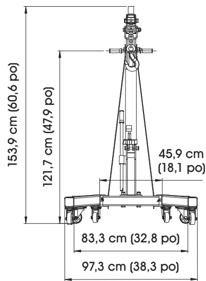
VUE ARRIÈRE
