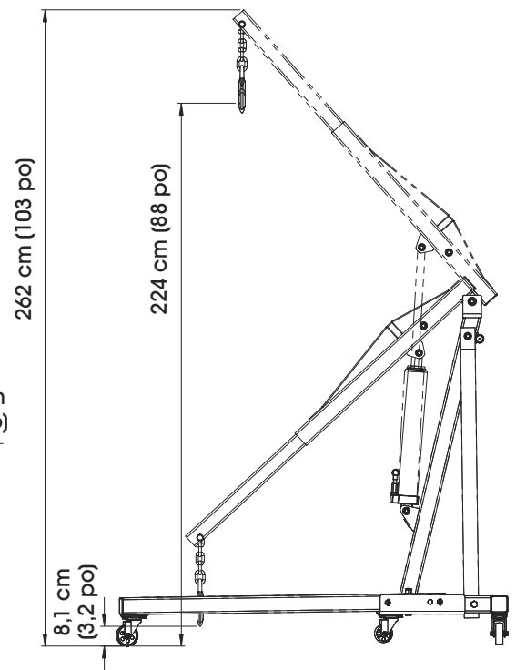
ÉLÉVATION
