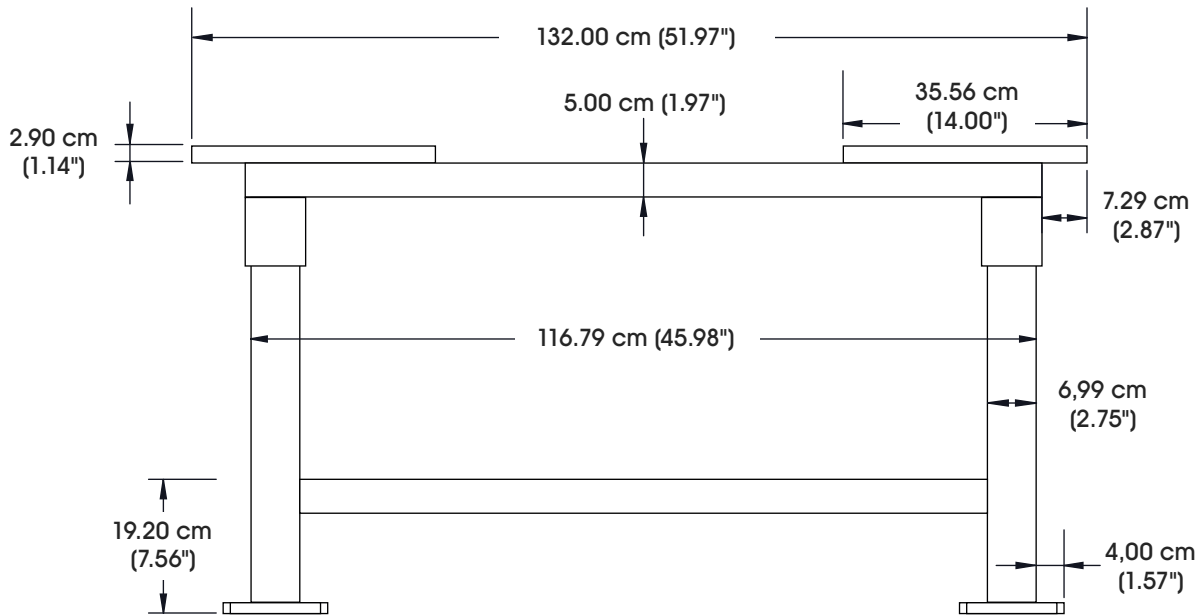
VISTA LATERAL
