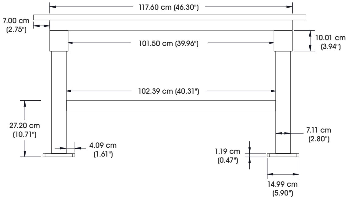
VISTA LATERAL
