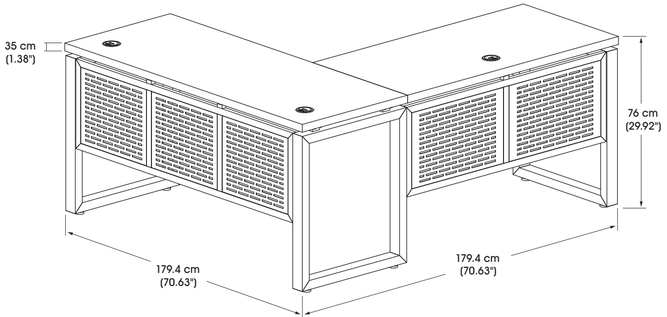
VISTA EXTERIOR
