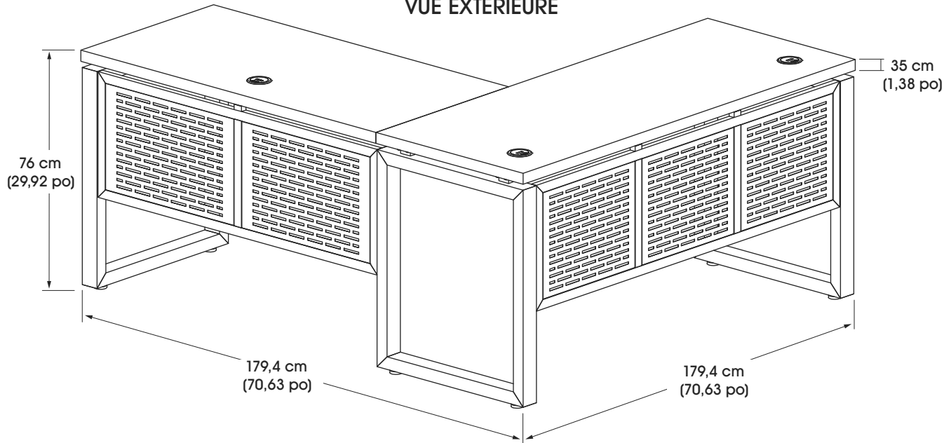
VUE EXTÉRIEURE
